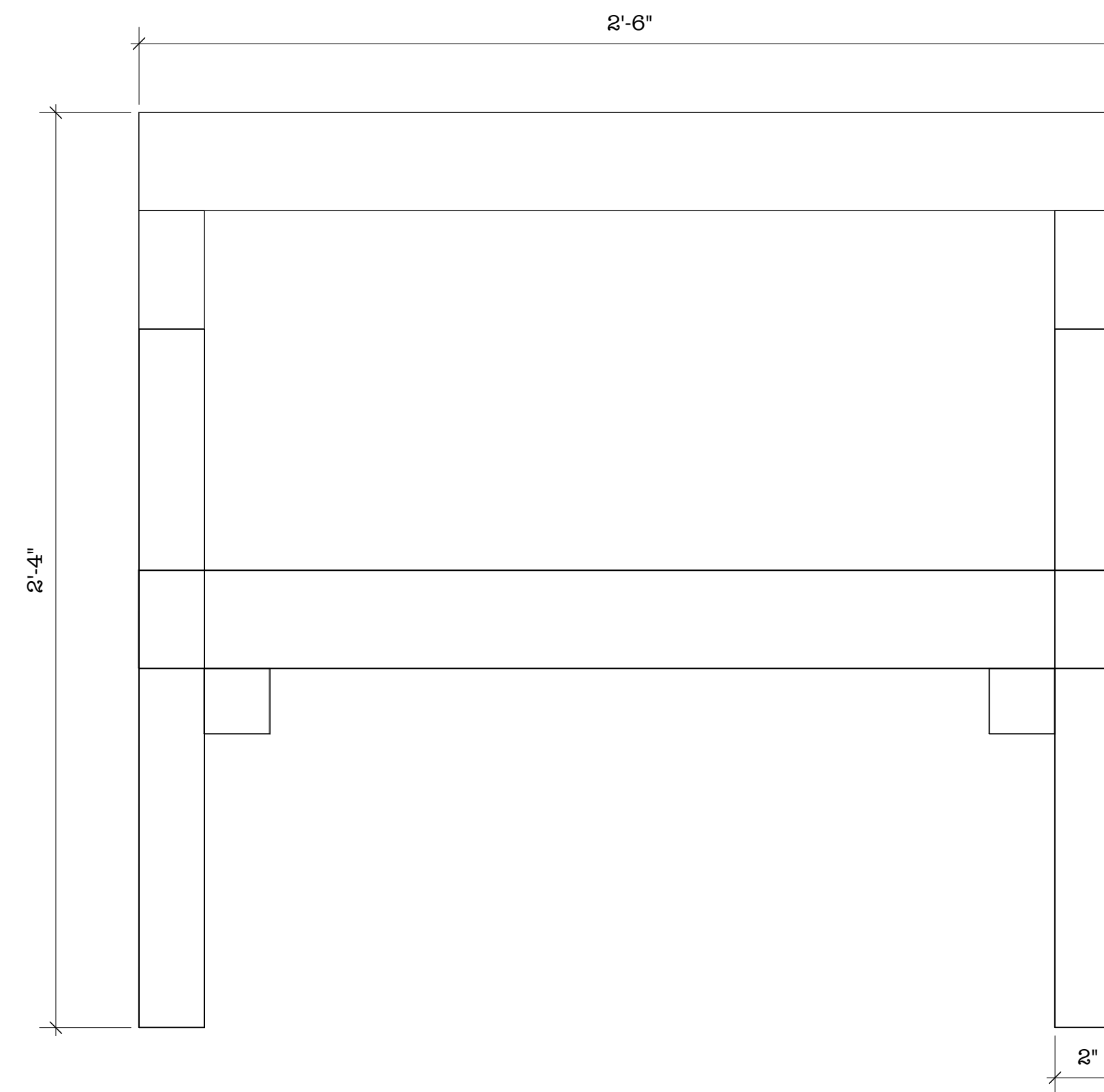
4 Left Scale: 3" = 1'-0"
