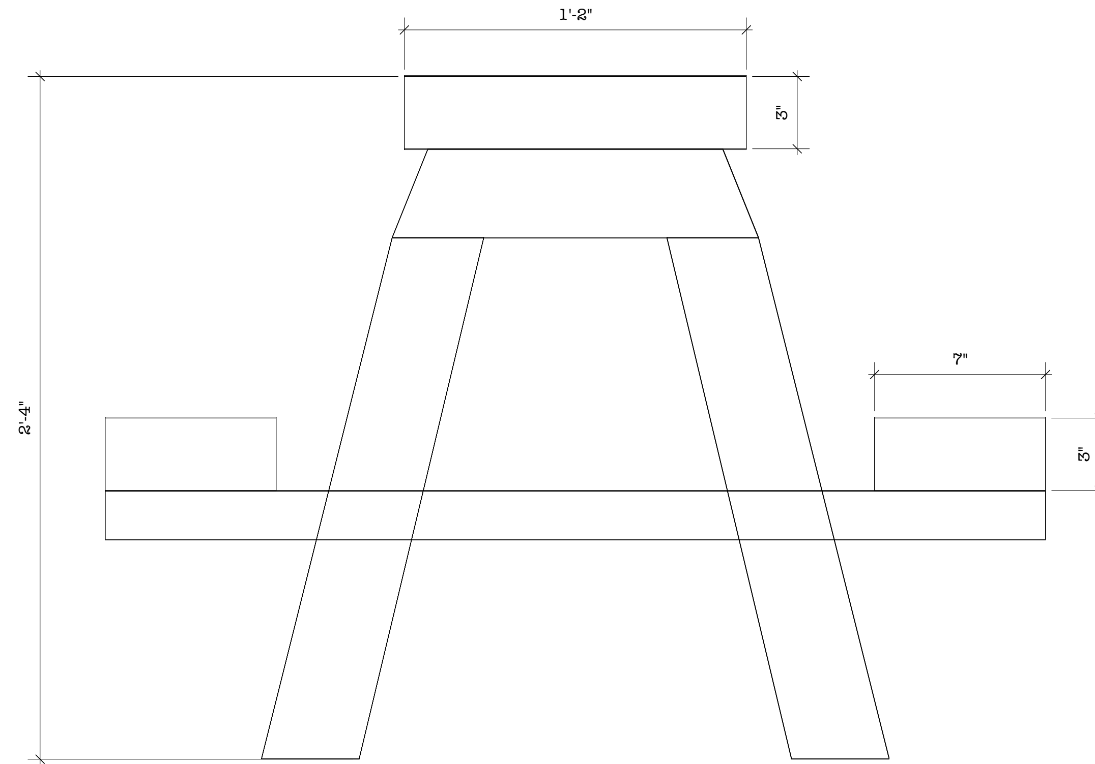
3 Front Scale: 3" = 1'-0"
